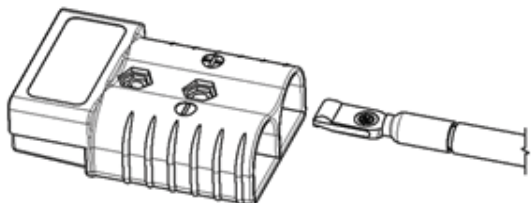
Montaggio del contatto cablato nella custodia Assembly of wired contact into housing
